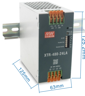
(XTR-480-xxLA)
